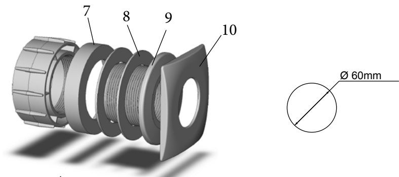
Assemblage sur paroi coque Prefabricated polyester pool assembly Montaje piscina prefabricada de poliester
