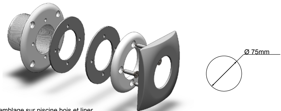
Assemblage sur piscine bois et liner Wooden pool with liner assembly Montaje piscina madera con liner
