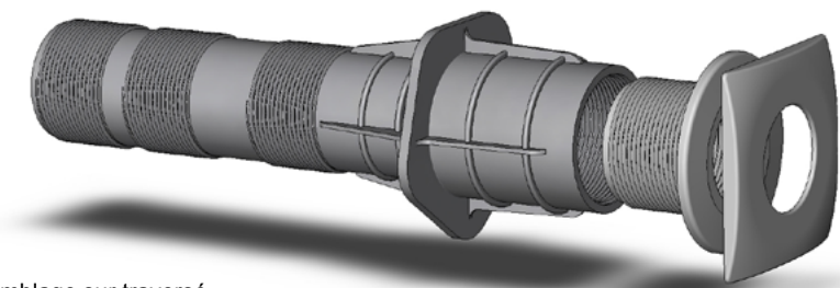
Assemblage sur traversé Assembly with threaded wall conduit Montaje con pasamuros roscado
